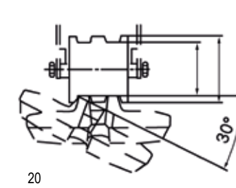
20 OPTIMALE KETTENFÜHRUNG
