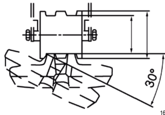
OPTIMALE KETTENFÜHRUNG
